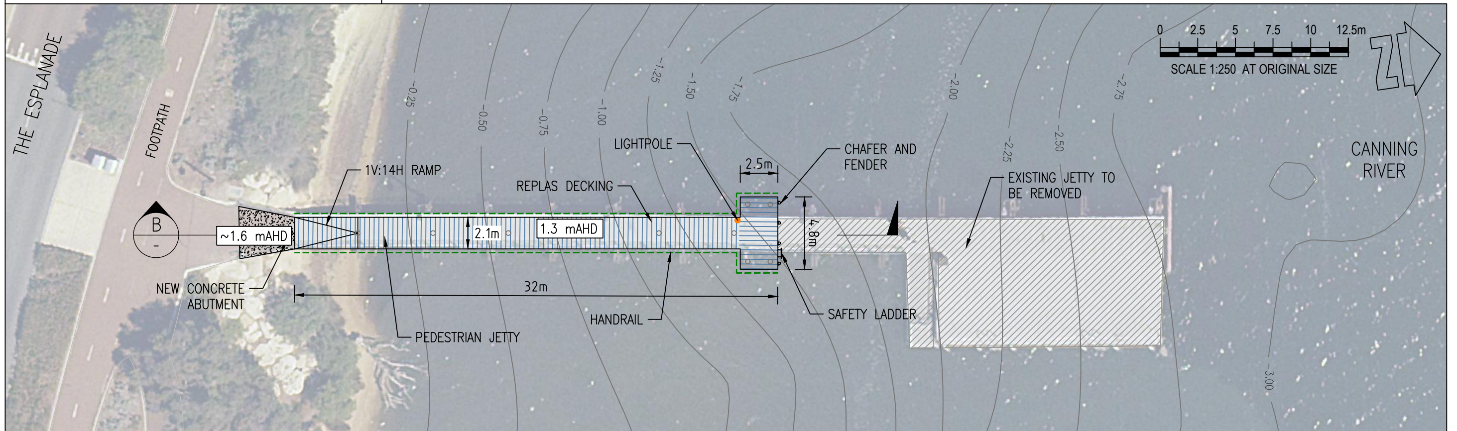
JETTY PLAN 1:250
