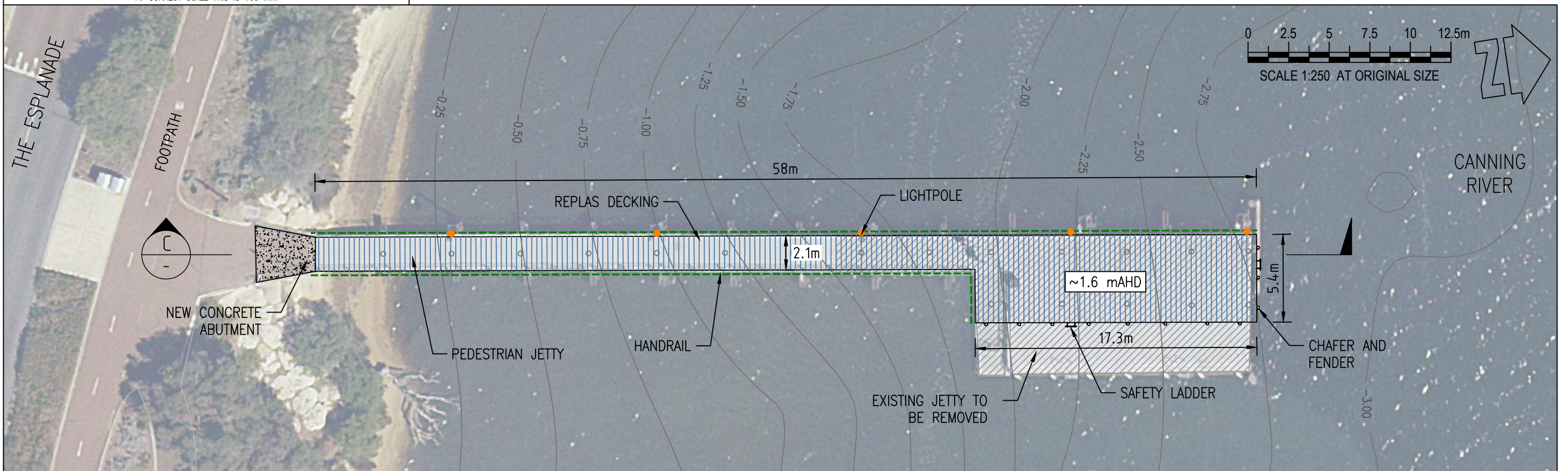
JETTY PLAN 1:250
