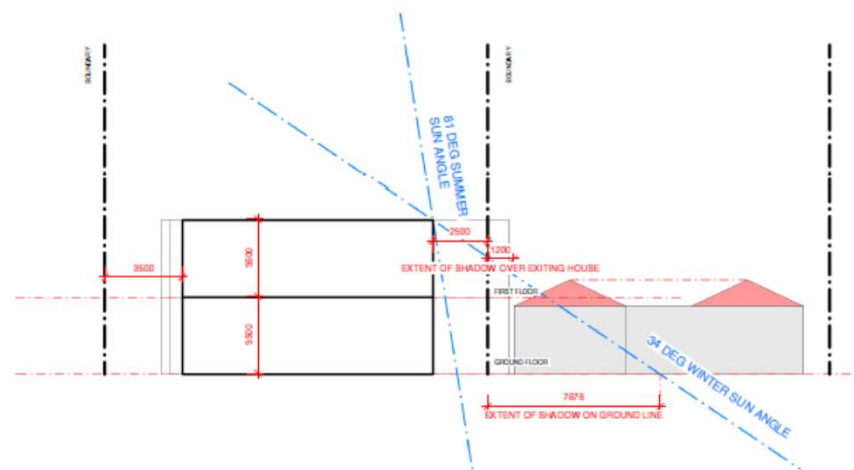
Section 1 1 : 100
